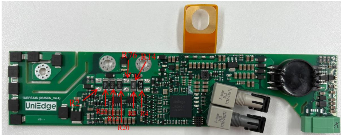
图 9- 1 门极电阻位置指示图
