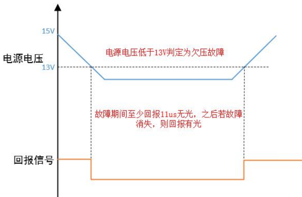
图 6- 3 欠压故障回报信号
